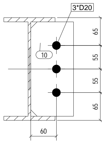
B - B 1:5
