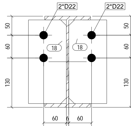
B - B 1:5
