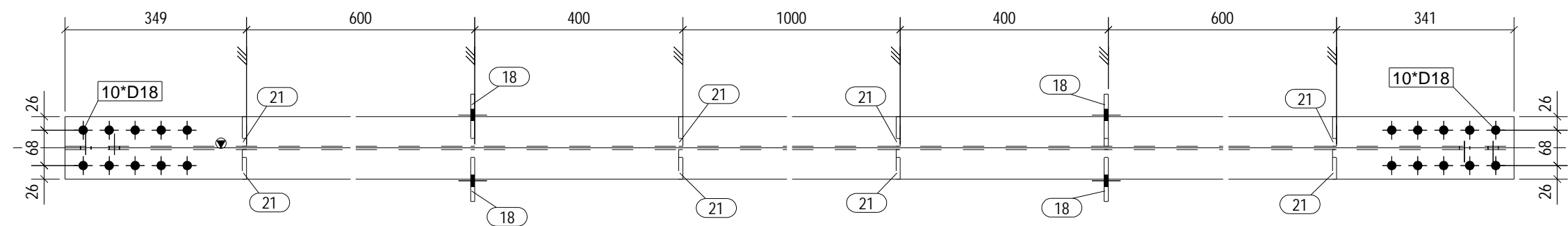
A - A 1:10
