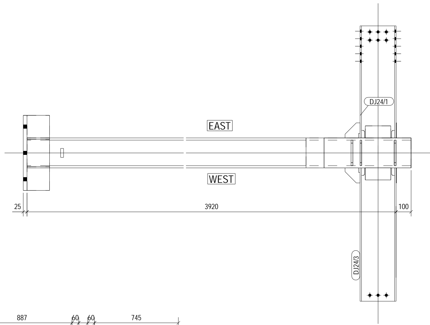
A - A 1:15
