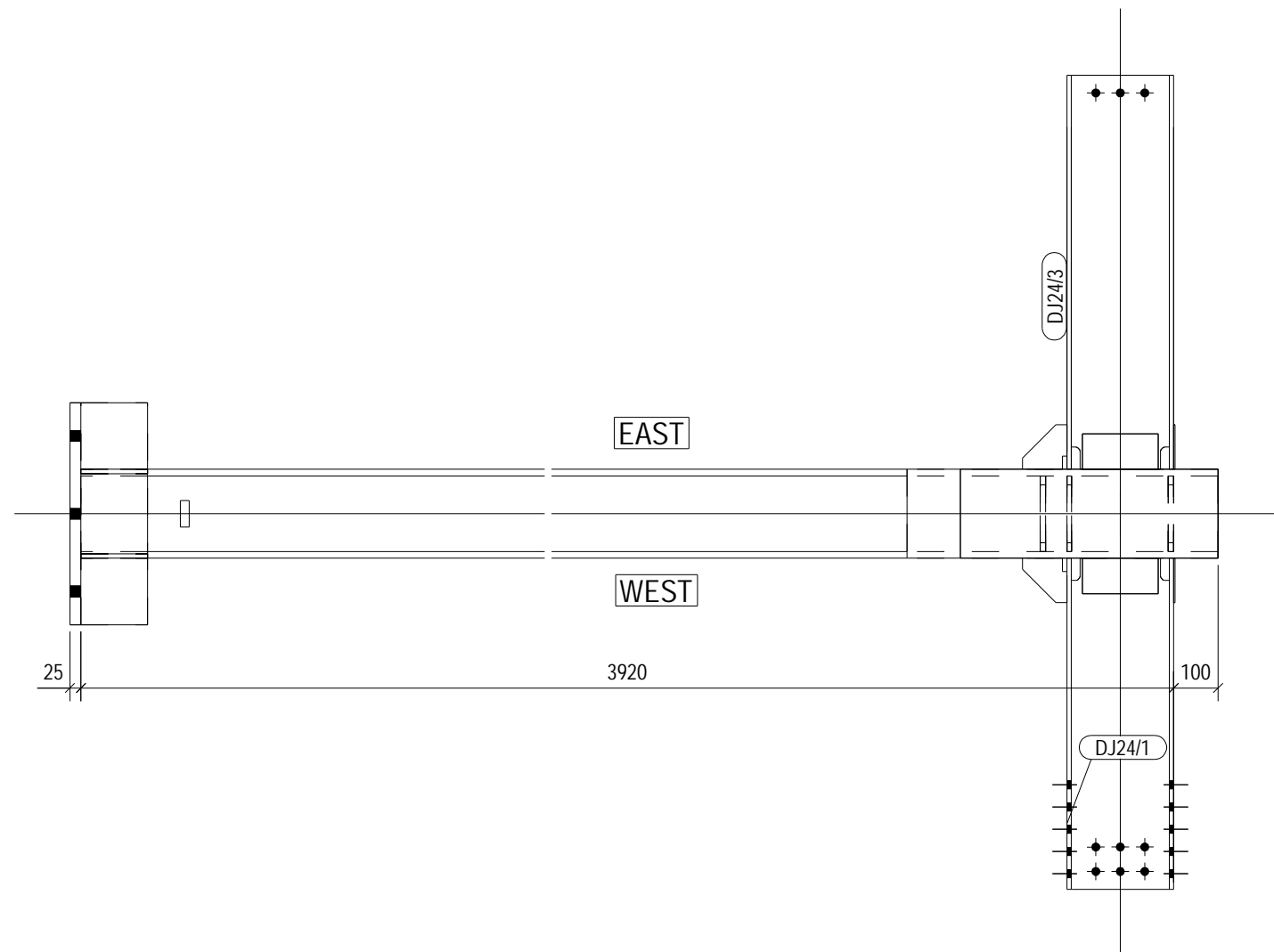
A - A 1:15
